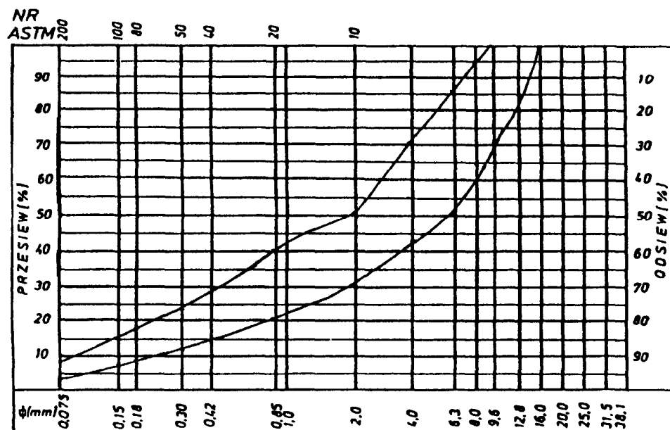
Rys. 1. Krzywe graniczne uziarnienia mieszanki mineralnej 0÷16, 0÷12,8 mm do warstwy ścierniej z betonu asfaltowego dla KR 1-2 Rys. 2. Krzywe graniczne uziarnienia mieszanki mineralnej 0÷16 mm do warstwy wiążącej, wyrówna
