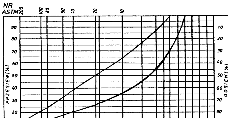
Rys. 1. Krzywe graniczne uziarnienia mieszanki mineralnej 0÷16, 0÷12,8 mm do warstwy ścierniej z betonu asfaltowego dla KR 1-2 Rys. 2. Krzywe graniczne uziarnienia mieszanki mineralnej 0÷16 mm do warstwy wiążącej, wyrówna
