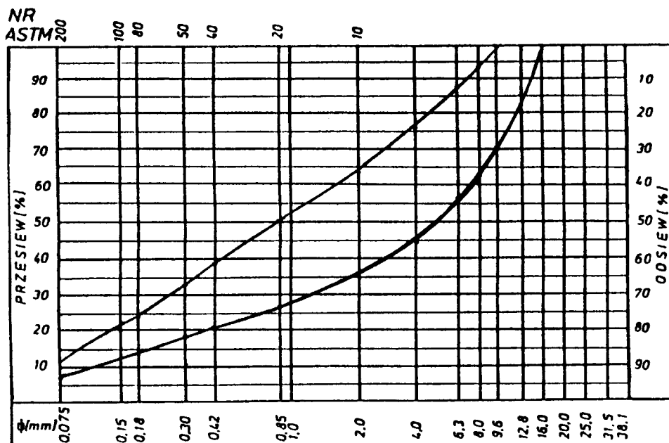
Rys. 1. Krzywe graniczne uziarnienia mieszanki mineralnej 0+16, 0+12,8 mm do warstwy ściernicowej z betonu asfaltowego dla KR 1-2
