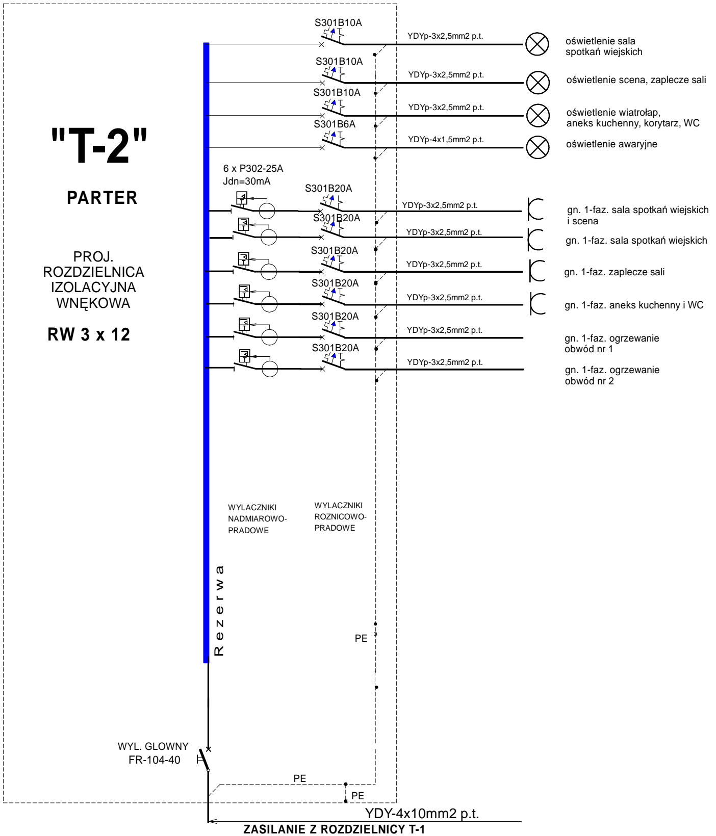
ROZDZIELNICA IZOLACYJA WNEKOWA RW - 3x12
