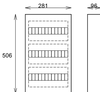
ROZDZIELNICA IZOLACYJA WNEKOWA RW - 3x12
