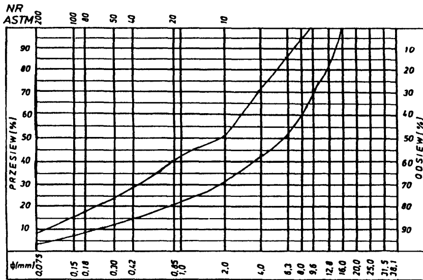
Rys. 1. Krzywe graniczne uziarnienia mieszanki mineralnej 0+16, 0+12,8 mm do warstwy ścieralnej z betonu
